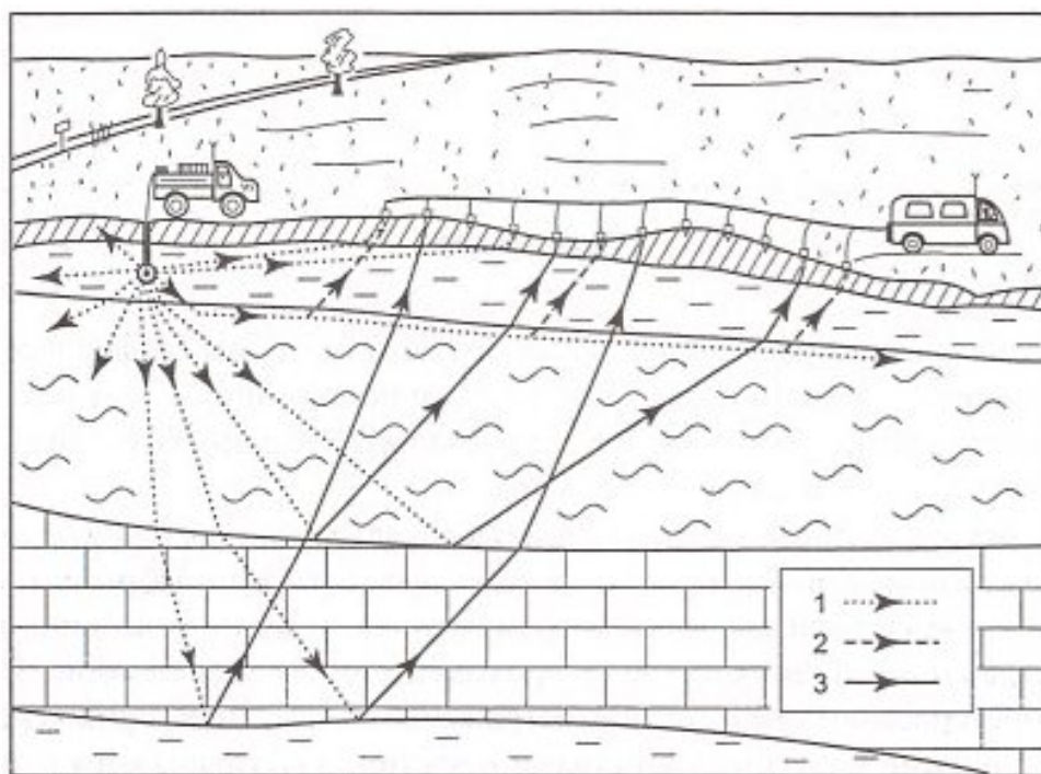
Рис. 3. Сейсмические наблюдения
