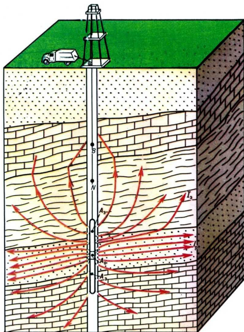
Рис. 4. Исследование скважины
