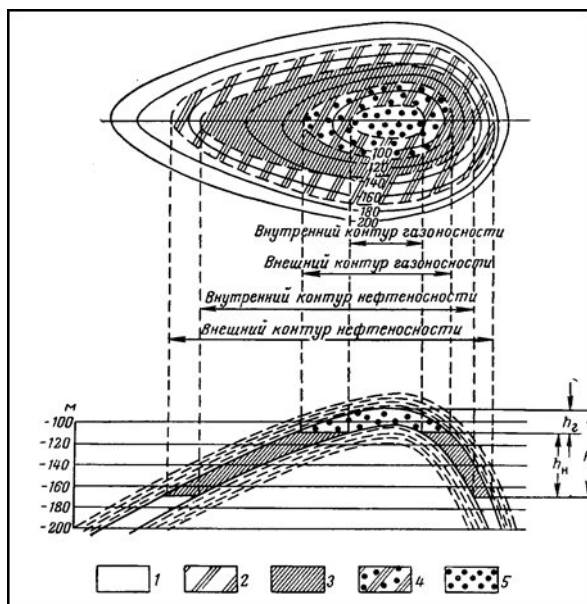
Рис. 2. Элементы залежи
