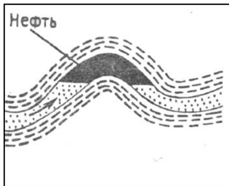
Рис. 1. Антиклинальная структура
